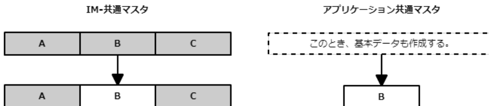
有効化された場合の新旧データ構造の変化
