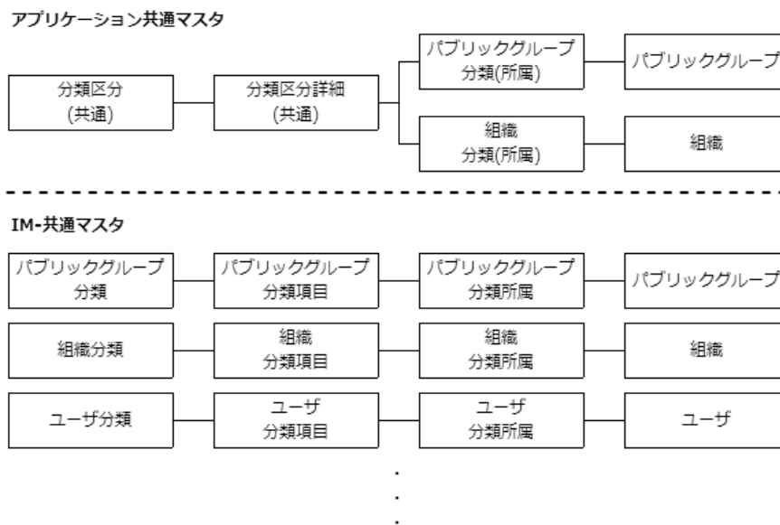
分類の構成の相違点
